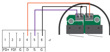
PI00 PCB1 & PI00 PCB2
