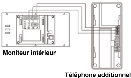
Schéma de branchement pour SOFIA 657
