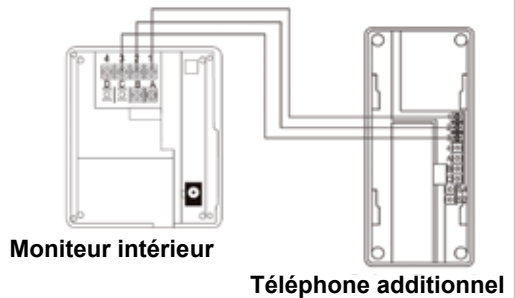
Schéma de branchement pour SOFIA : 600 / 620 / 811-2 G / 811C-2 G
