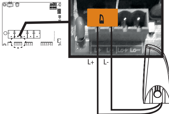
CARD (CONTROL BOX)
